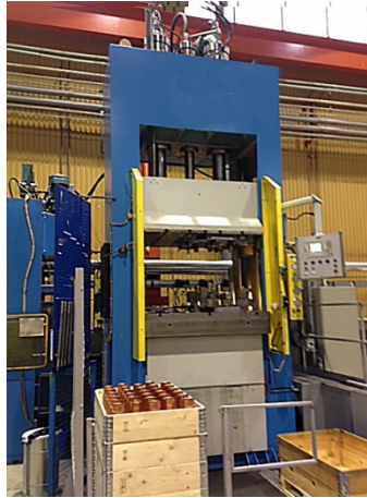
Här en liknande press som AGAB har till salu, men med enklare utförande - även denna på 5000kN presskraft.
